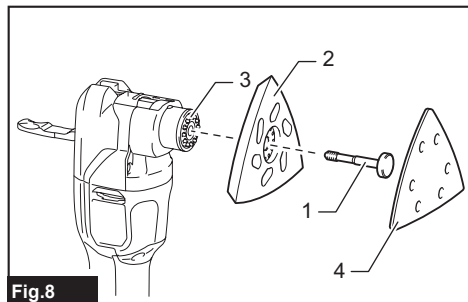
Fig.8 ► 1. Boulon de retenue 2. Outil d'application (patin de ponçage) 3. Flasque d'outil 4. Papier abrasif
