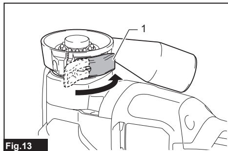
Fig.13 ► 1. Clamp lever
