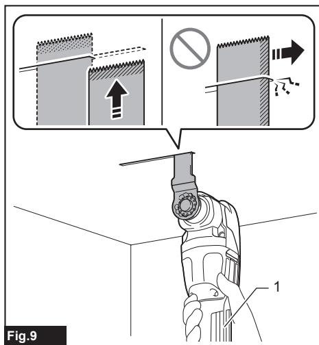
Fig.9 ► 1. Poignée (prise isolée)
